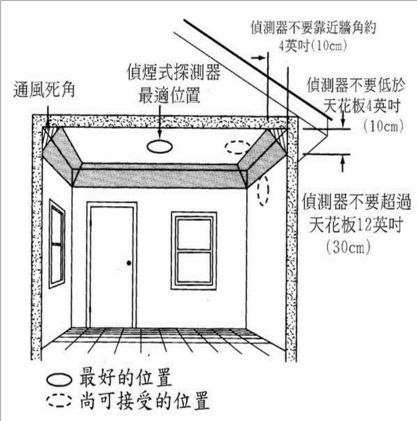
火災(偵煙)警報器安裝位置示意圖
